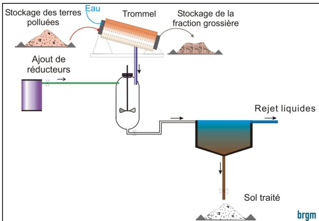
Figure 10 – Schéma de principe de l'oxydation chimique
