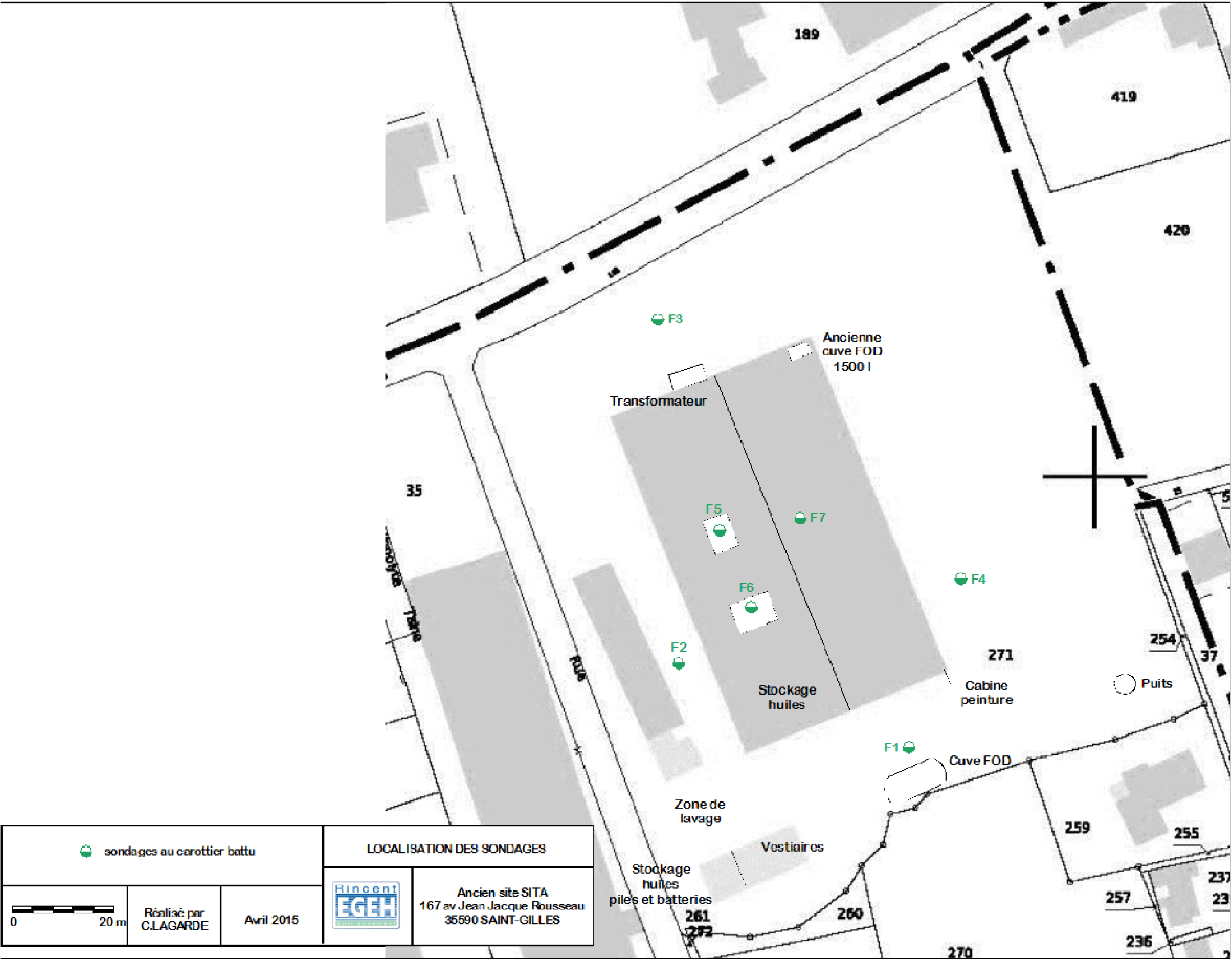
Figure 2 – Schéma d’implantation des sondages de mars 2015
